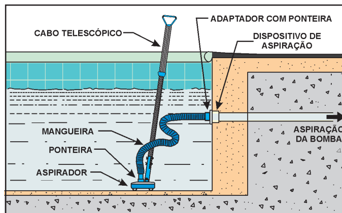
Exemplo 2: Instalação do aspirador no dispositivo de aspiração
